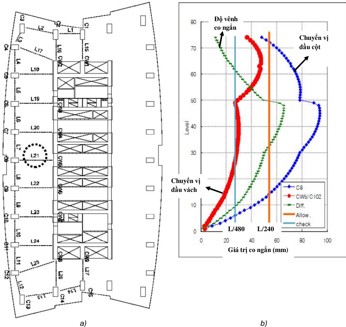
Hình 2. Hotel tower – a) Mặt bằng tầng điển hình; b) Giá trị co ngấn của cột C8 và vách CW5 [7]
