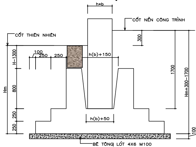
MÓNG CÁC TRỤC
