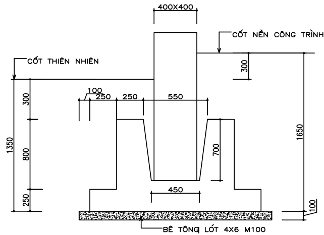
MÓNG SƯỜN TƯỜNG
