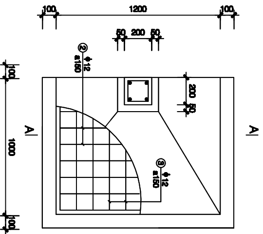
MẶT BẰNG MÔNG M1
