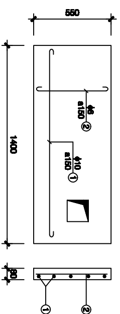
DAN D2 (1 CK)
