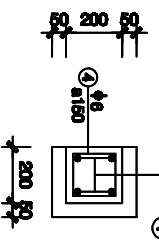
MẶT CẮT 1 - 1
