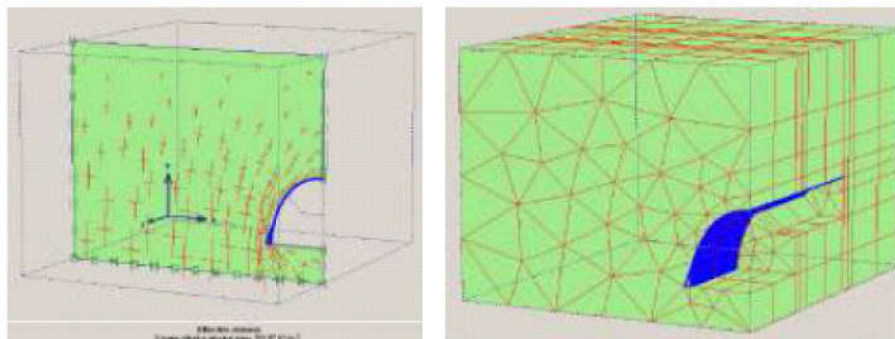
Phân bố các ứng suất hiệu quả quanh đường hầm trên một mặt phẳng vuông góc với trục hầm
