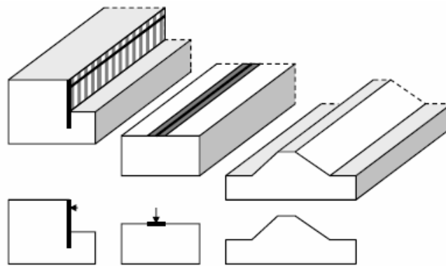
Hình 2.3. Các dạng bài toán sử dụng mô hình biến dạng phẳng AXI-SYMMETRY
