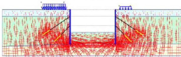
Hình 1.1: Phân tích bài toán hố đào bằng Plaxis 2D V8.5
