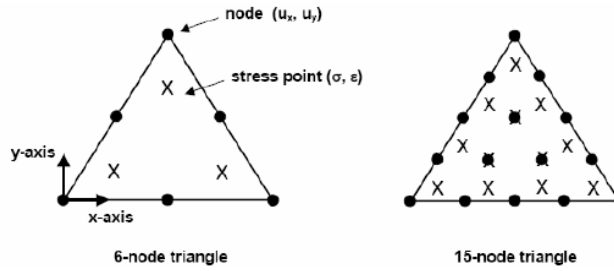
Hình 2.5. Phần tử tam giác 6 nút và 15 nút
